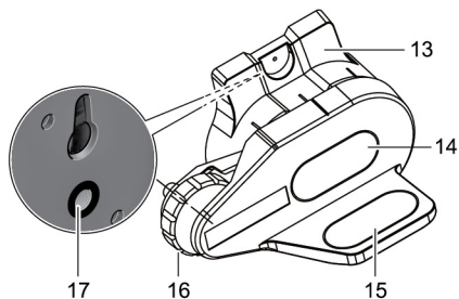
Рис. 2 Универсальный кронштейн
