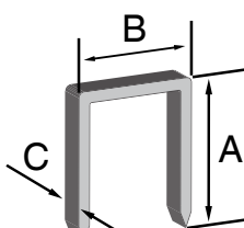
Параметры скобы
